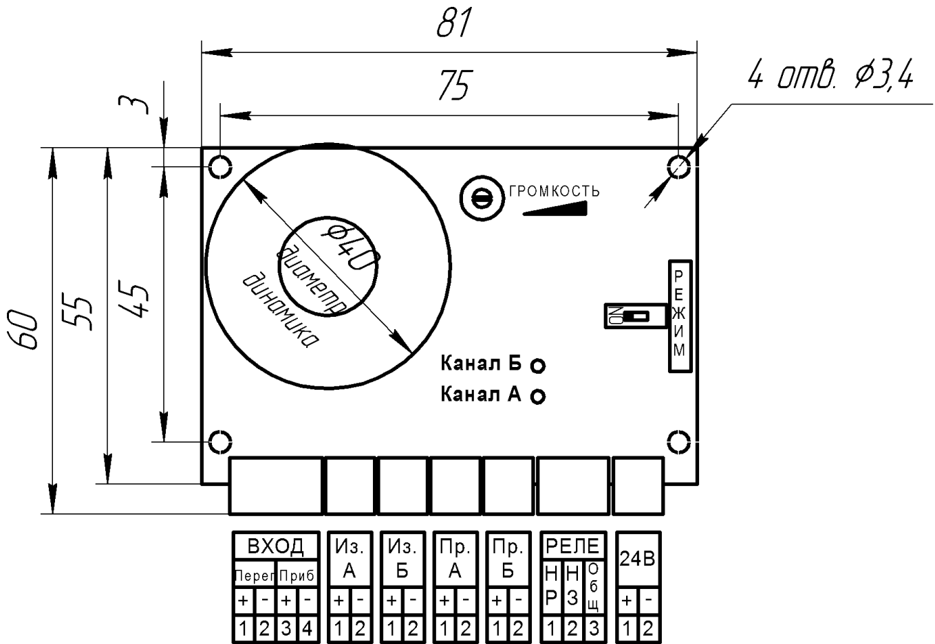
Рис.2. Габаритные и установочные размеры
