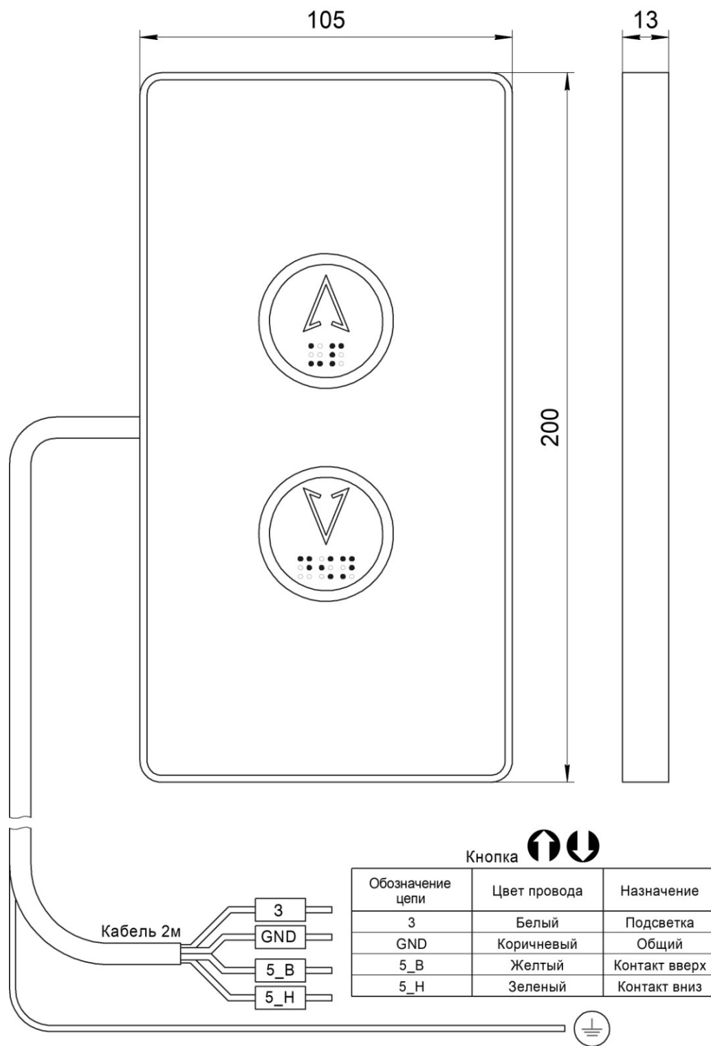
Рис.1 Внешний вид, габаритные и установочные размеры Вызывного поста МАЛАХИТ НШЕК.468381.084
