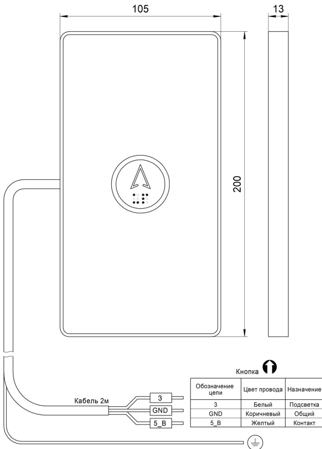
Рис.1 Внешний вид и габаритные размеры Вызывного поста МАЛАХИТ НШЕК.468381.082
