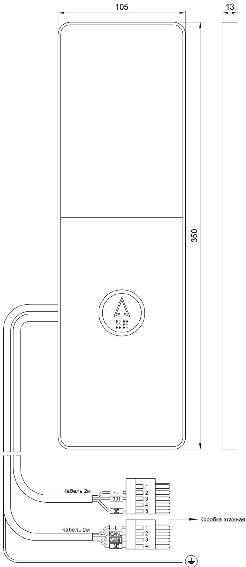
Рис.1 Внешний вид, габаритные и установочные размеры Вызывного поста МАЛАХИТ (ШК) НШЕК.468381.129
