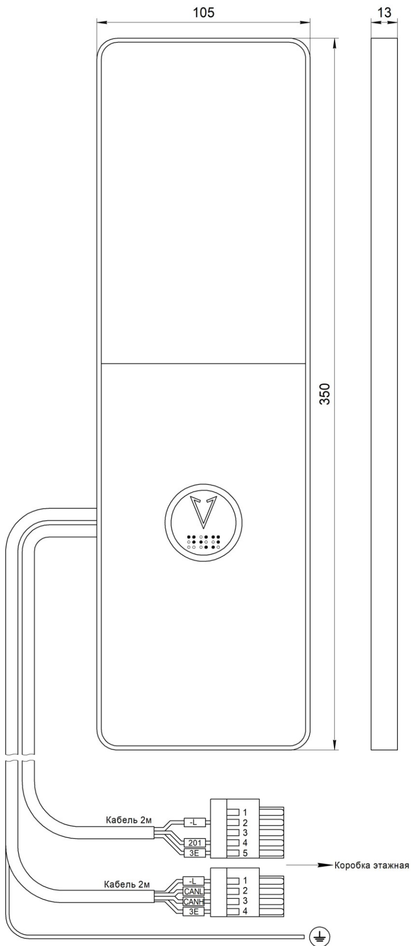
Рис.1 Внешний вид, габаритные и установочные размеры Вызывного поста МАЛАХИТ (ШК) НШЕК.468381.129-01
