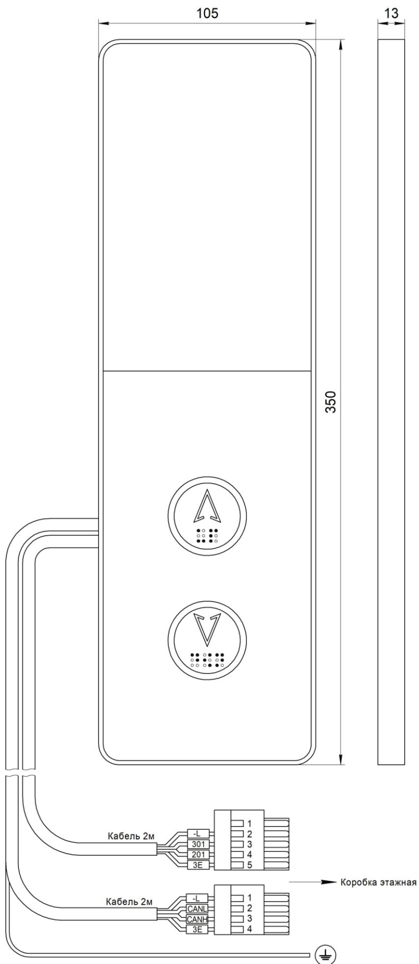
Рис.1 Внешний вид, габаритные и установочные размеры Вызывного поста МАЛАХИТ (ШК) НШЕК.468381.130
