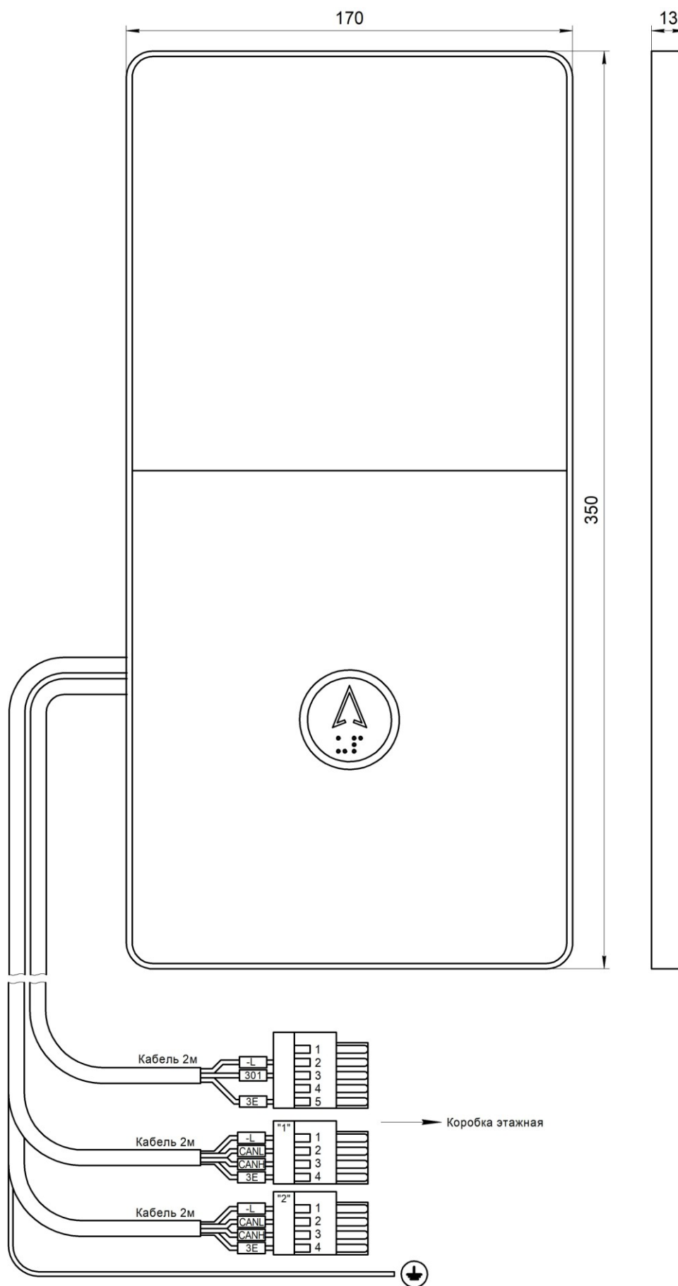
Рис.1 Внешний вид, габаритные и установочные размеры Вызывного поста МАЛАХИТ (ШК) НШЕК.468381.131
