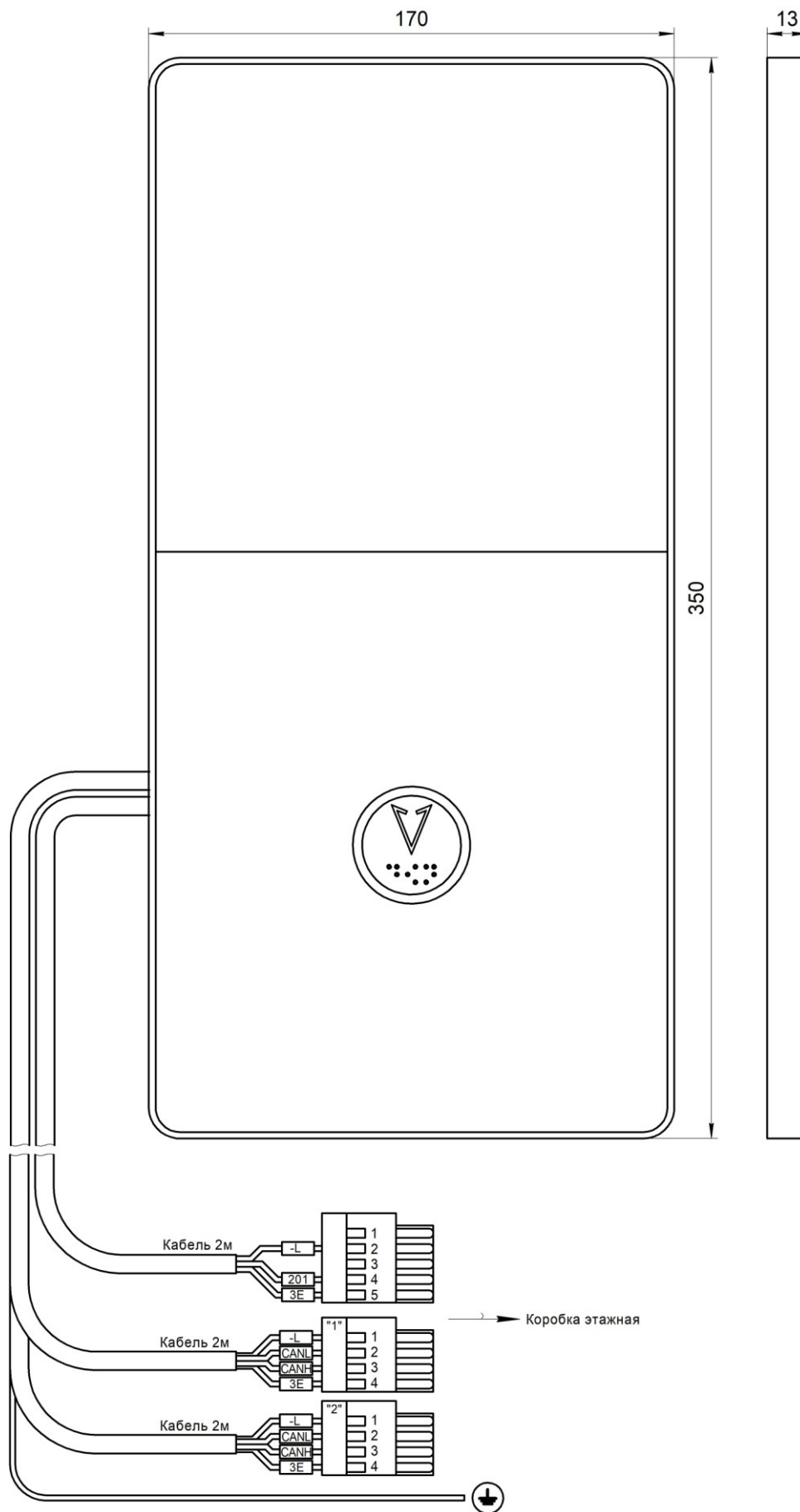
Рис.1 Внешний вид, габаритные и установочные размеры Вызывного поста МАЛАХИТ (ШК) НШЕК.468381.131-01
