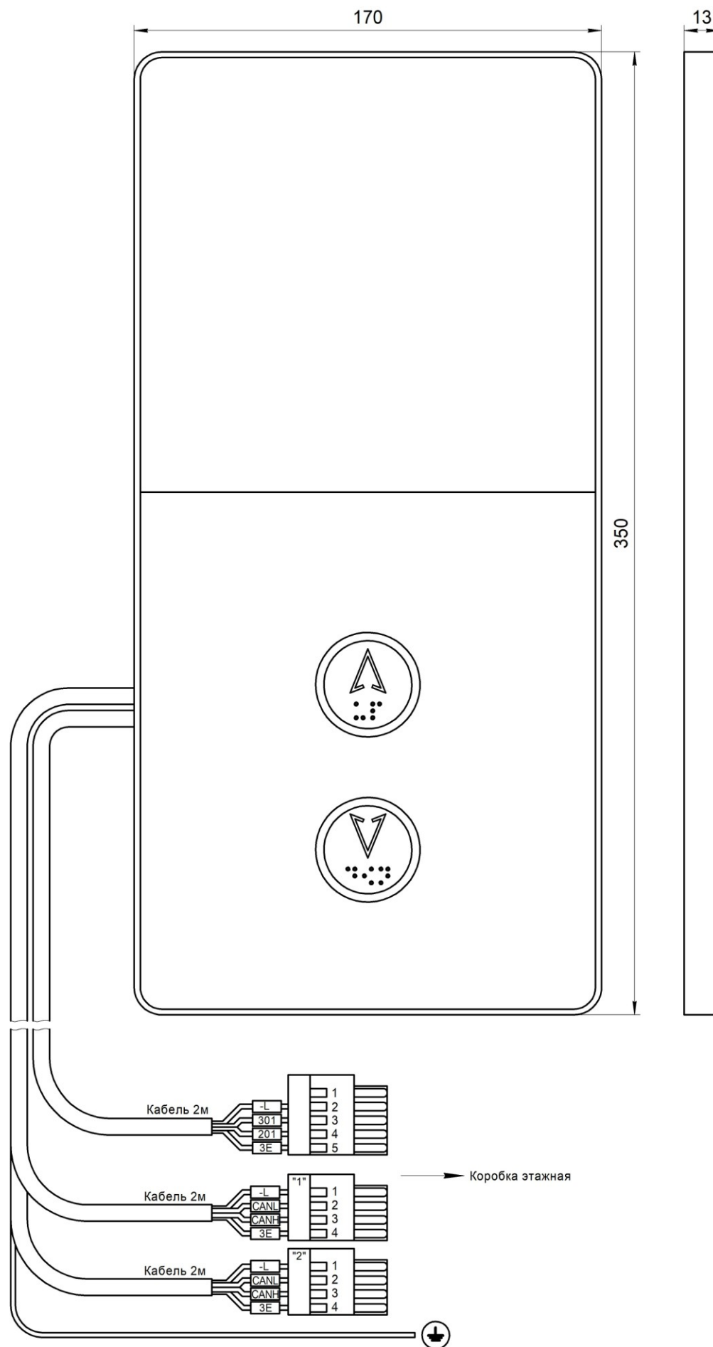
Рис.1 Внешний вид, габаритные и установочные размеры Вызывного поста МАЛАХИТ (ШК) НШЕК.468381.132
